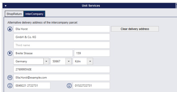
Figure 155 – IntercompanyService
